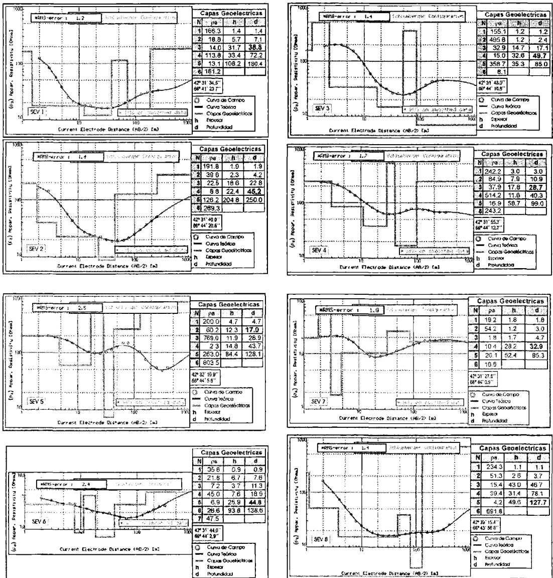
Figura 3. Capas geoelectricas correspondientes a cada uno de los Sondeos Eléctricos Verticales y profundidad estimada del basamento.
