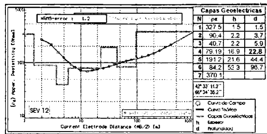
Figura 4. Capas geoelectricas correspondientes a cada uno de los Sondeos Eléctricos Verticales y profundidad estimada del basamento.
