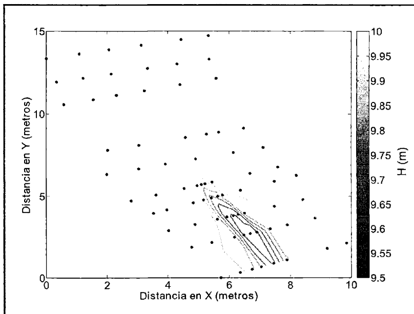
Figura 2. Registro original de mediciones de topografía en función de las coordenadas espaciales. Superpuestas se presentan las curvas de nivel obtenidas de la realización de la grilla inicial.
