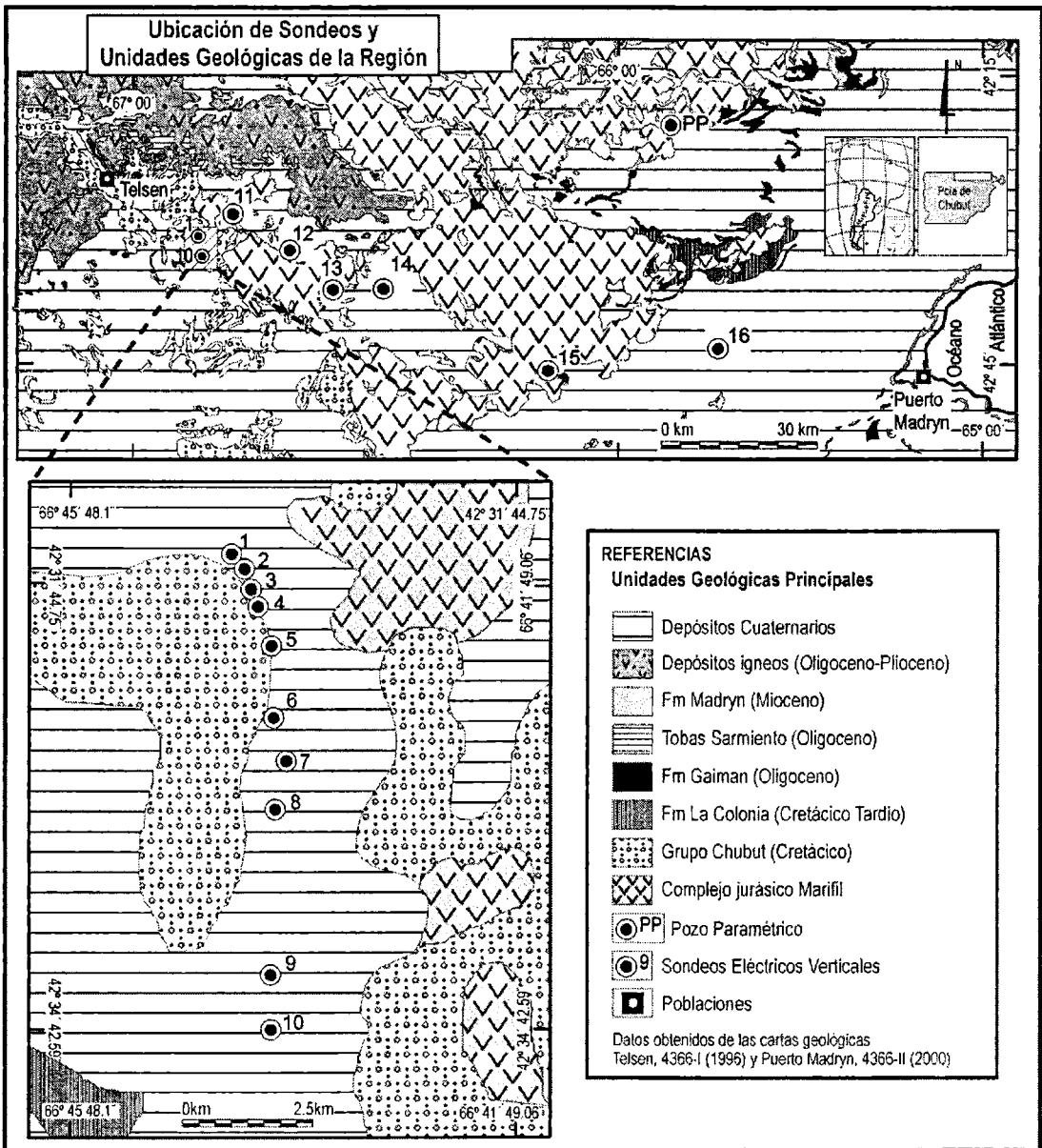
Figura 1: Área de estudio y unidades geológicas asociadas. Ubicación de los puntos de sondeo geoelectrónico y del pozo de exploración paramétrico.
