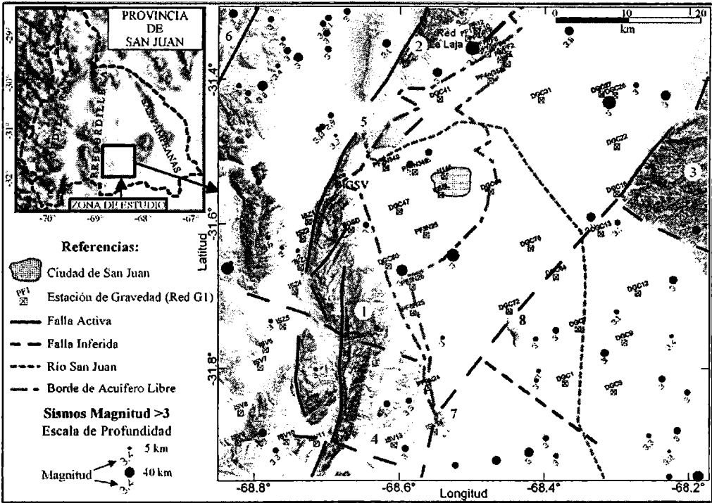
Figura 1. Ubicación de la zona de estudio. Modelo digital del terreno (SRTM 90m) con fallas activas y límite de acuífero libre. Cuadrados: puntos fijos de la Red G1. Círculos negros: epicentros de terremotos M>3, período 01-11-2000 a 15-11-2004 (escala de profundidades en referencias) 1: Sa. Chica de Zonda; 2: Sa. de Villicum; 3: Sa. Pie de Palo; 4: Qda. La Flecha; 5: Dique de Ullum; 6: Precordillera Central; 7: Co. Valdivia; 8: Co. Barboza.
