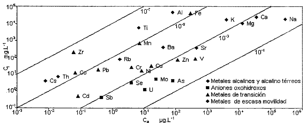
Figura 2. Concentración promedio de elementos en el agua subterránea ( C_a ) versus la del loess ( C_l ).
