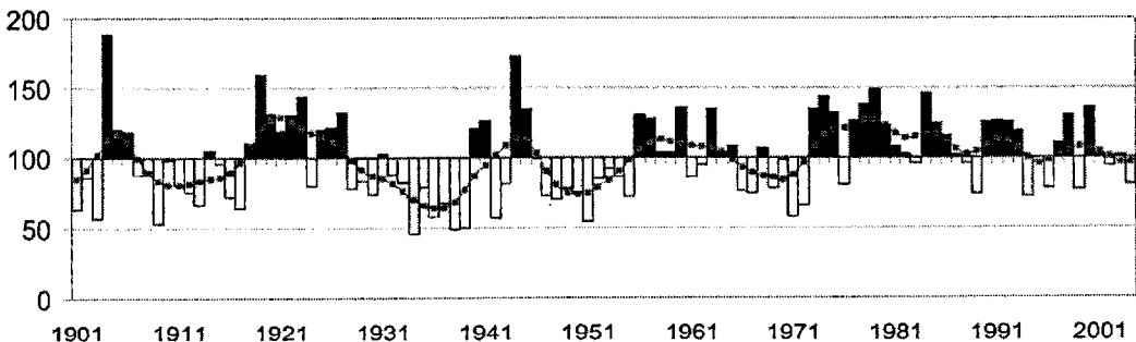
Figura 1. Valores porcentuales del índice regional de precipitación estival P(t) para el COA (barras verticales) y suavizado gaussiano de 9 términos (línea con círculo) (Hoel, 1964).
