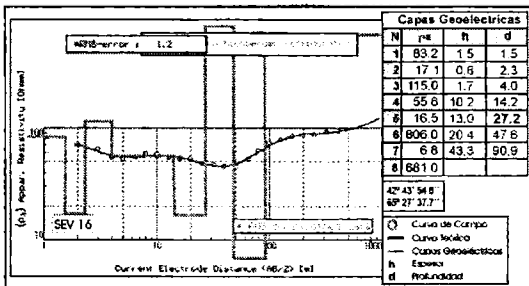
Figura 4. Capas geoelectricas correspondientes a cada uno de los Sondeos Eléctricos Verticales y profundidad estimada del basamento.
