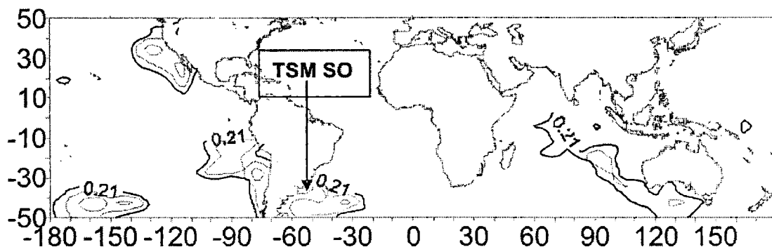
Figura 3. Áreas de correlación significativa para el intervalo de confianza de 95% entre la precipitación estival en el COA y la TSM (Hadley Center) en el período 1904-1994. TMS SO: área de mayor varianza explicada, entre 30°-40°S y desde la costa de Sudamérica hasta 40°O aproximadamente.
